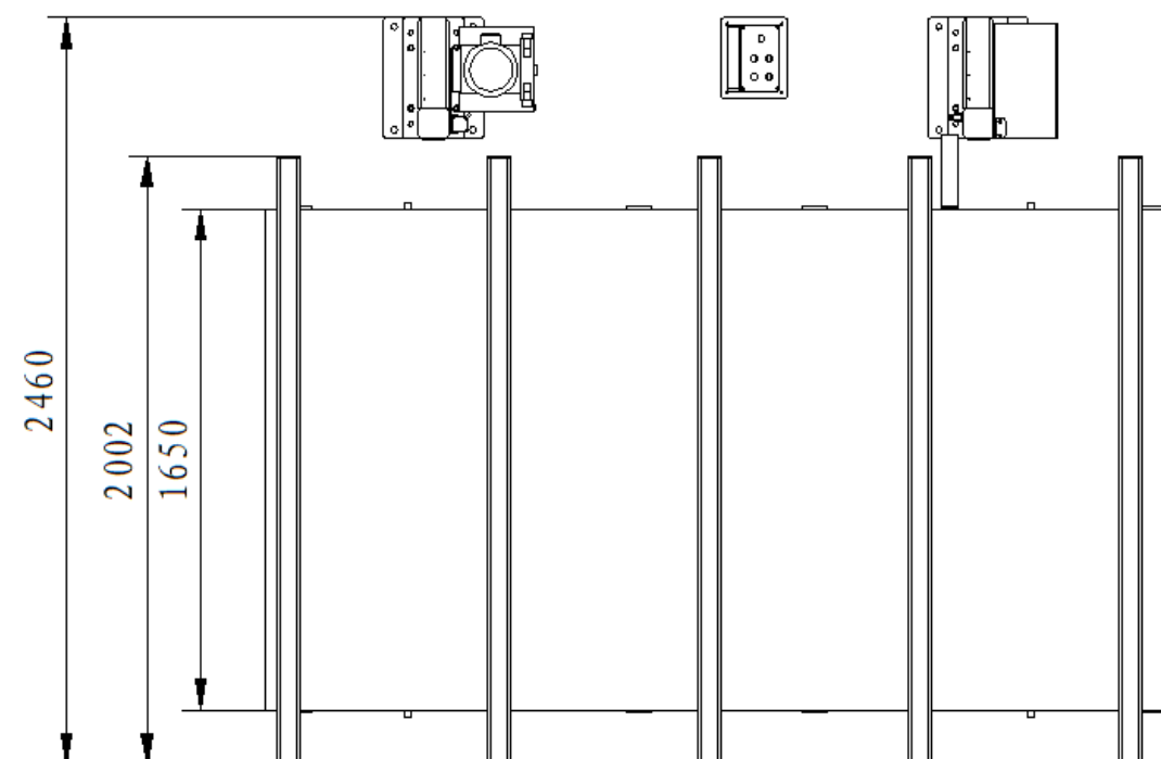
KHA-2710布局图
